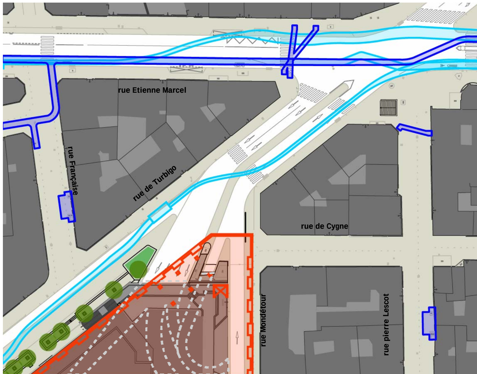
Turbigo - rue du Cygne : les galeries techniques
